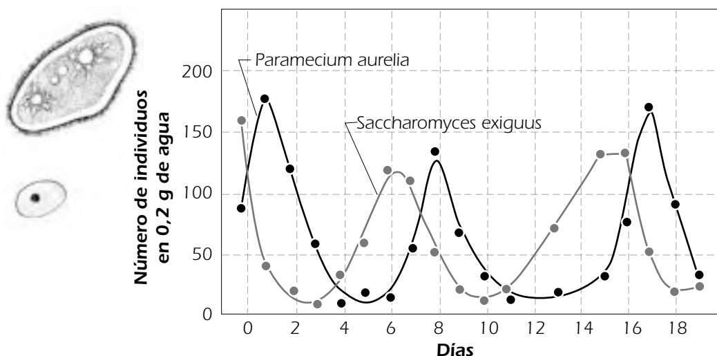
Modelo Presa-Depredador
